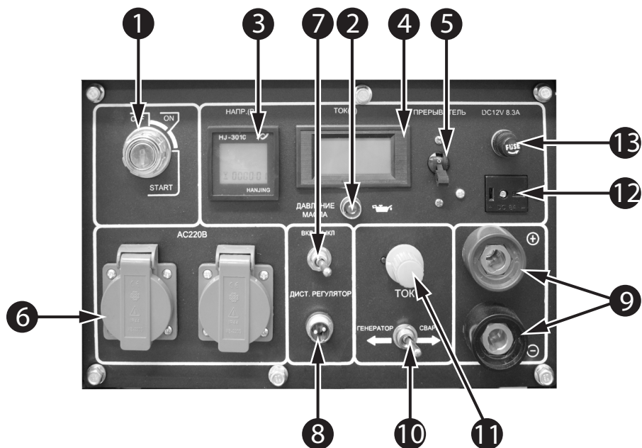
Рис. 2 Панель управления
