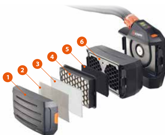
Защита от твердых частиц и газа
